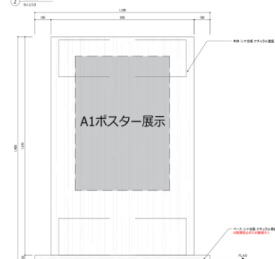
③ 正面図 S=1/20
