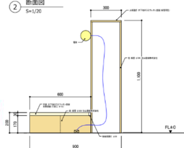
② 断面図 S=1/20
